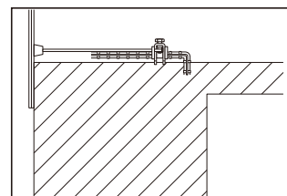
②土間止めでの使用に
