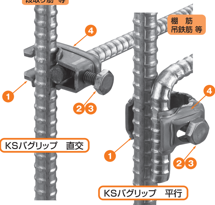
KSバグリップ直交型
