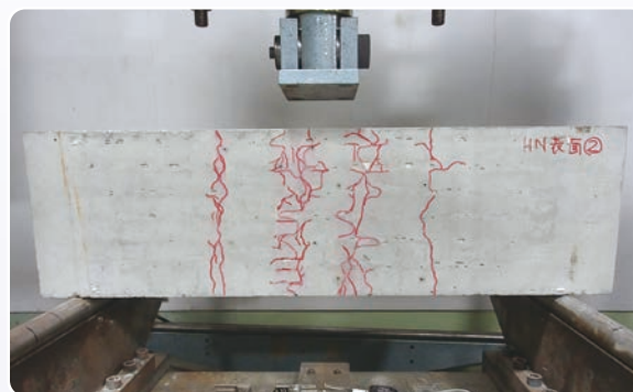
ハイパーネットSS 表面敷設 ひび割れ4本
