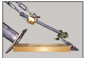
◎栈木等を利用して押し引き同時使用※
